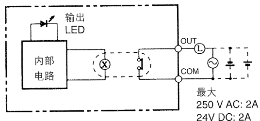
CQM1-OC224
