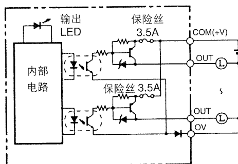
CQM1-OD214
