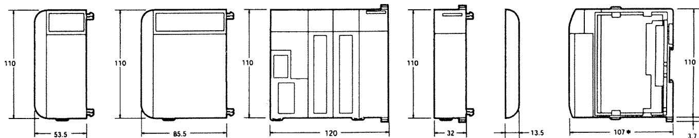
ID/IA/OC/OD/OA□ 端板 (通信单元和专用 I/O 单元)
