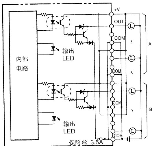
CQM1-OD213
