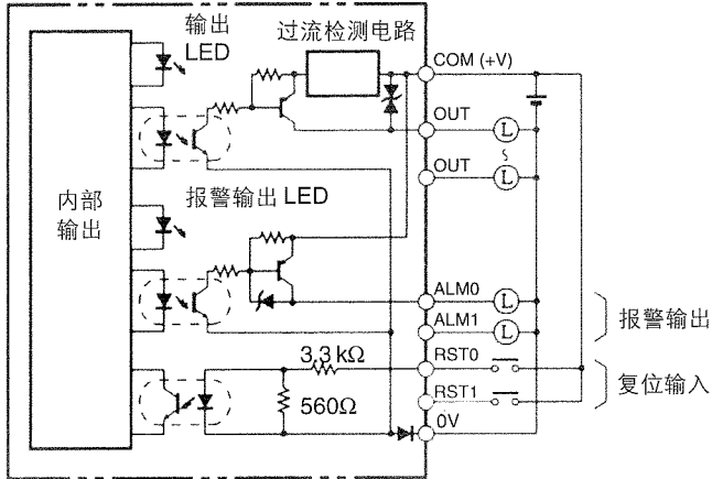
CQM1-OD215
