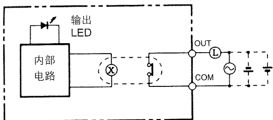
CQM1-OC221
